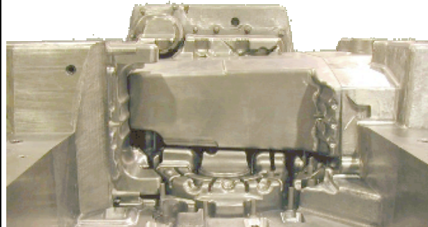
Druckgussformen
