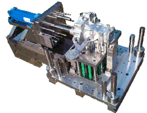
Kokillen
